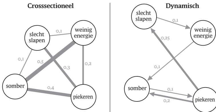
FIGUUR 2 Voorbeelden van een crosssectioneel en dynamisch netwerk. In het crosssectionele netwerk is somberheid het meest centrale symptoom (0,1 + 0,4 + 0,5 = 1,0), omdat dat de sterkste verbindingen heeft met de andere symptomen. In het dynamische netwerk heeft piekeren de hoogste uitgaande centraliteit, want dit symptoom voorspelt het sterkst andere symptomen (0,25 + 0,2 = 0,45). Het symptoom met de grootste ingaande centraliteit is hier somberheid (0,1 + 0,2 = 0,3), omdat dit symptoom het sterkst voorspeld wordt uit andere symptomen.
